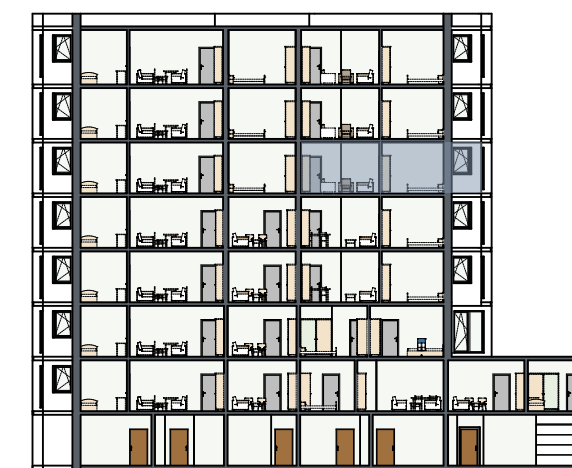
ŘEZ OBJEKTEM:
